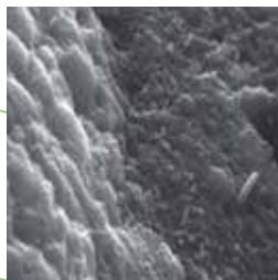
Bindmiddel KONKREA HPM 750F – veel dichtere structuur (schaal 7 µm)
